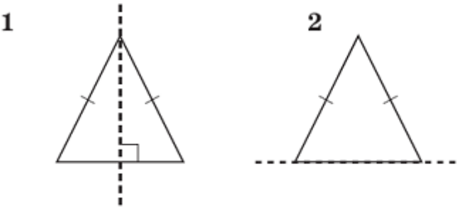
рівнобедрені трикутники
