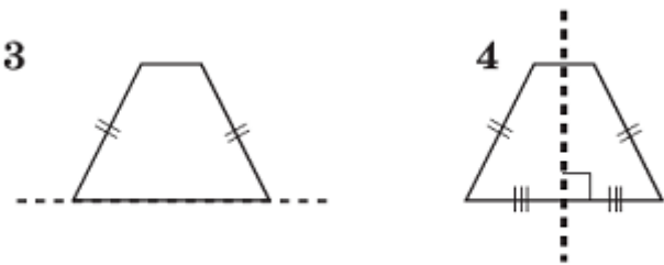
рівнобічні трапеції
